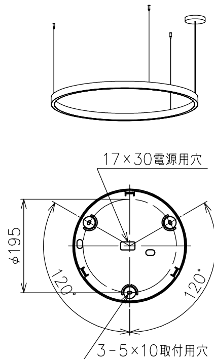
取付板詳細
